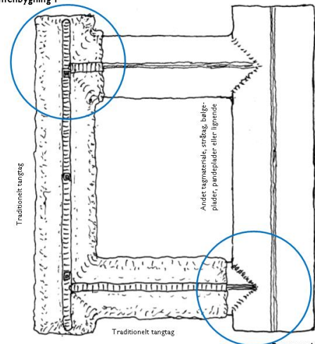
Sammenbygning 2
